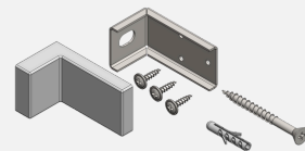
CONJUNTO DE FIJACIÓN A LA PARED
