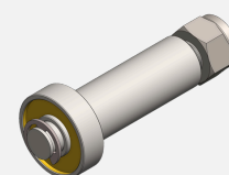
PINO M10 - PORCA M10 - ROLAMENTO - ANEL ELÁSTICO
