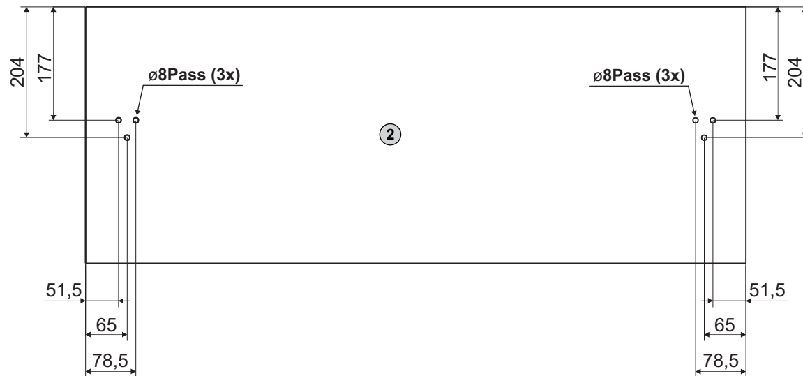
2 - Tampo Caixa/Tapa de la Caja/Box Top
